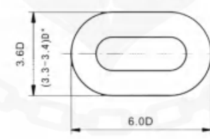
STUDLESS LINK=SL (无档链)
