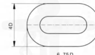
END LINK=E (末端链环)
