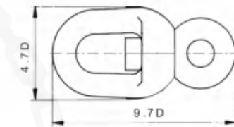
SWIVEL=SW (转环)
